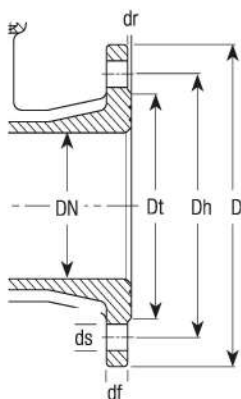
Otwory wg ISO 7005 część 2 (PN-EN 1092-2, DIN 2501)
