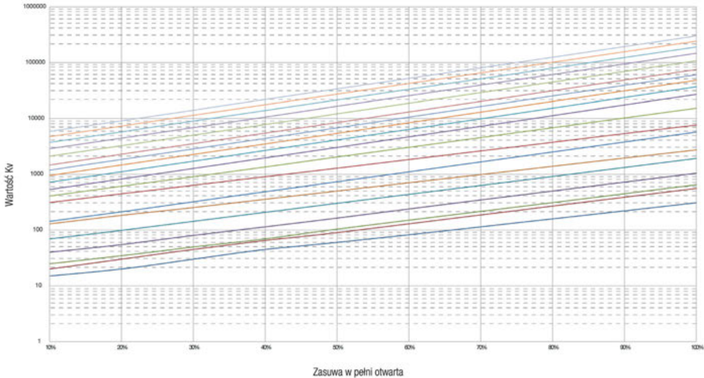
Wartość Kv dla zasuw klinowych DN40-1000
