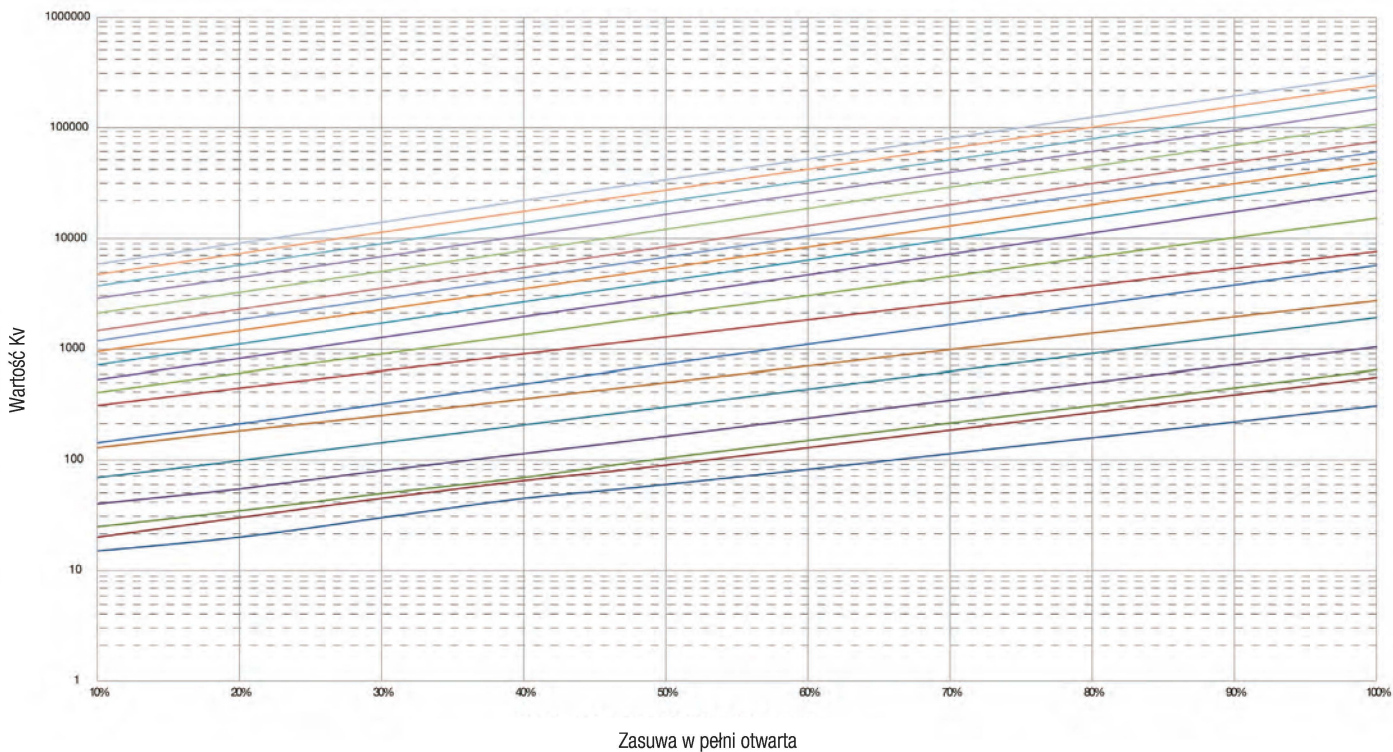
Wartość Kv dla zasuw klinowych DN40-1000
